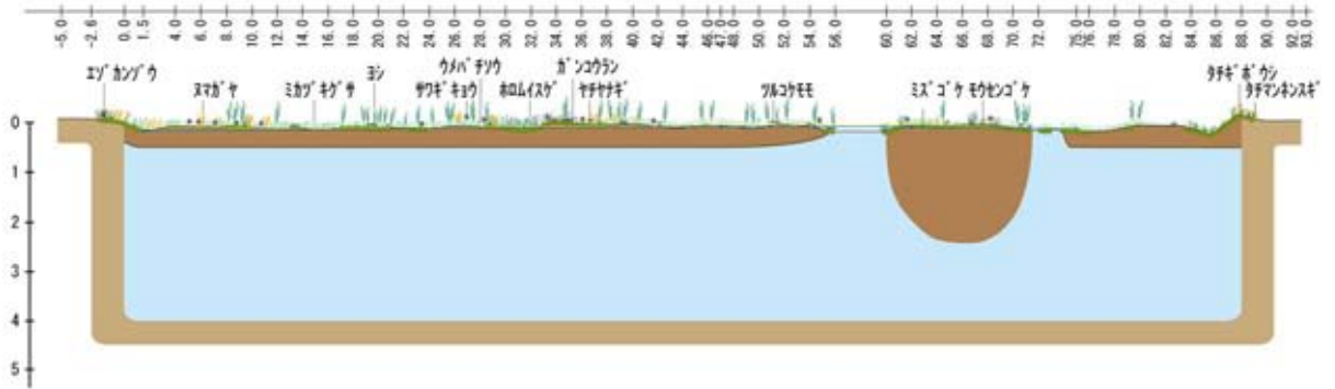
図 5-23 基盤構造と植生断面模式(浮島状の採掘跡地)
