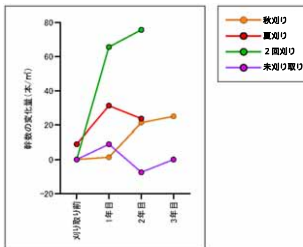
図 3-8 稈数の推移
